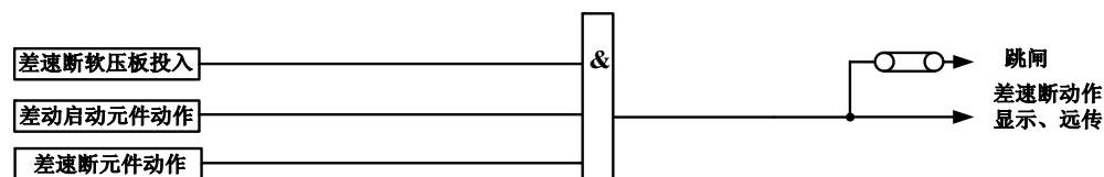
图 3-13 差动速断保护原理框图
