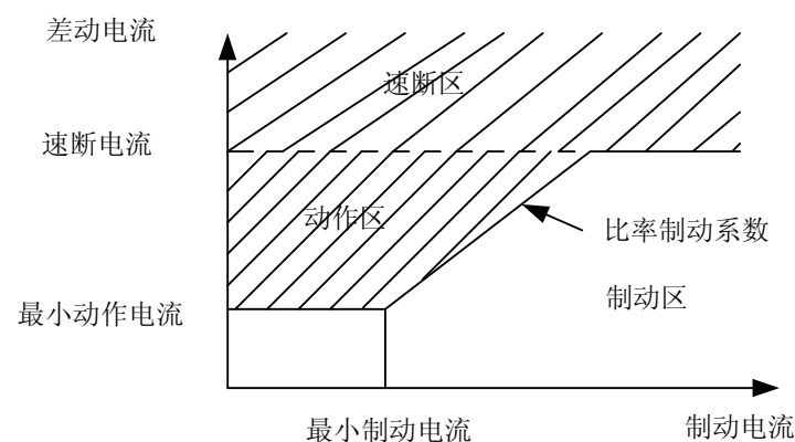
图 3-14 差动动作曲线
