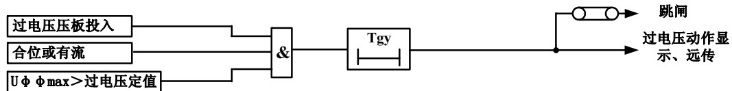
图 3-8 电动机装置过电压保护原理框图
