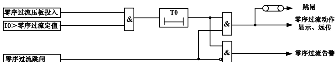
图 3-6 零序过流保护原理框图
