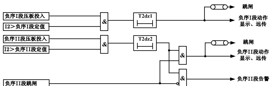
图 3-5 负序过流保护原理框图
