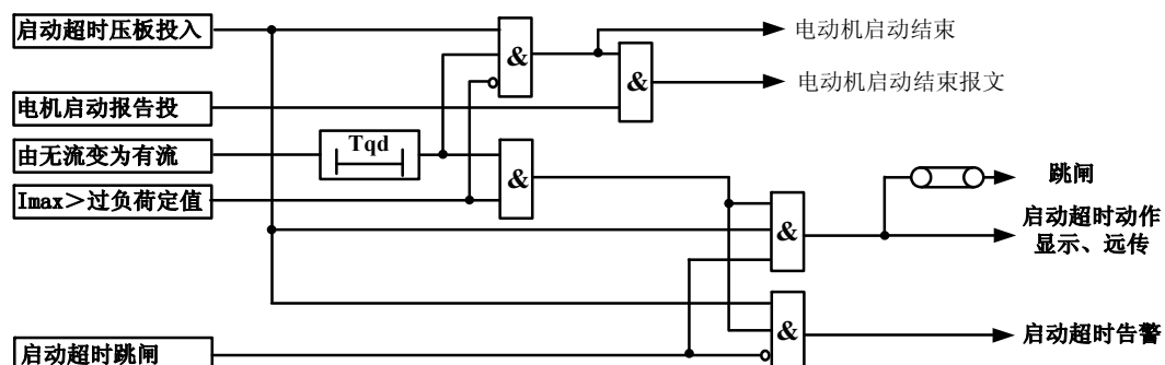
图 3-2 电动机启动超时保护原理框图
