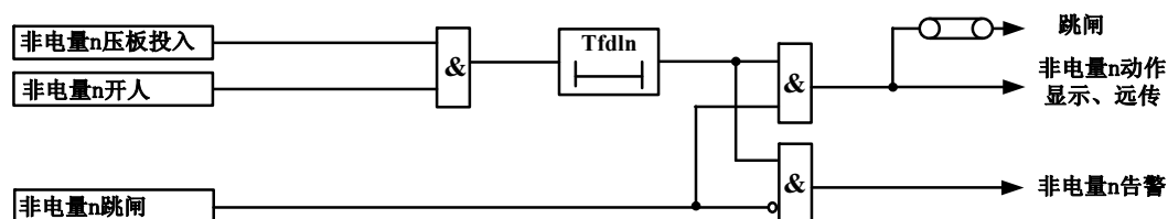
图 3-11 非电量保护原理框图
