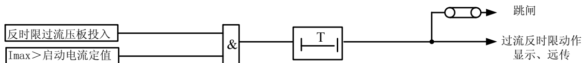
图 3-4 反时限过流保护原理框图
