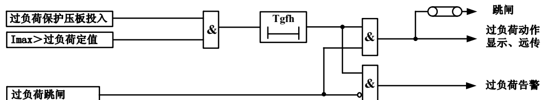
图 3-10 过负荷保护原理框图
