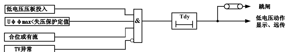
图 3-7 低电压保护原理框图
