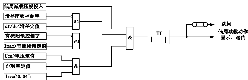
图 3-9 低周减载原理框图
